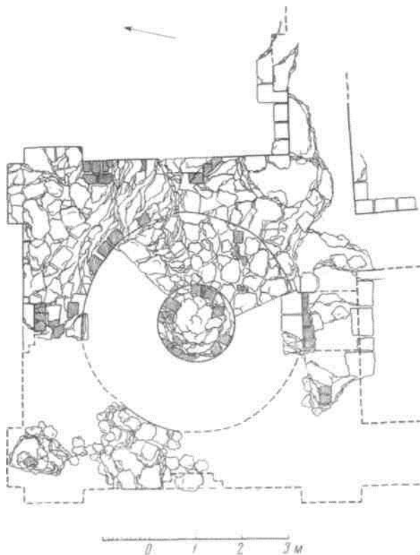
Рис. 3. Лестничная башня после раскопок. План
