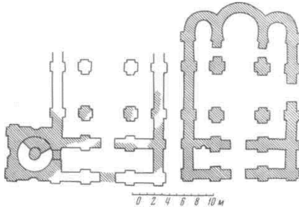
Рис. 5. Планы церкви Благовещения на Городище (1103 г.) и Николо-Дворищенского собора (1113 г.)
